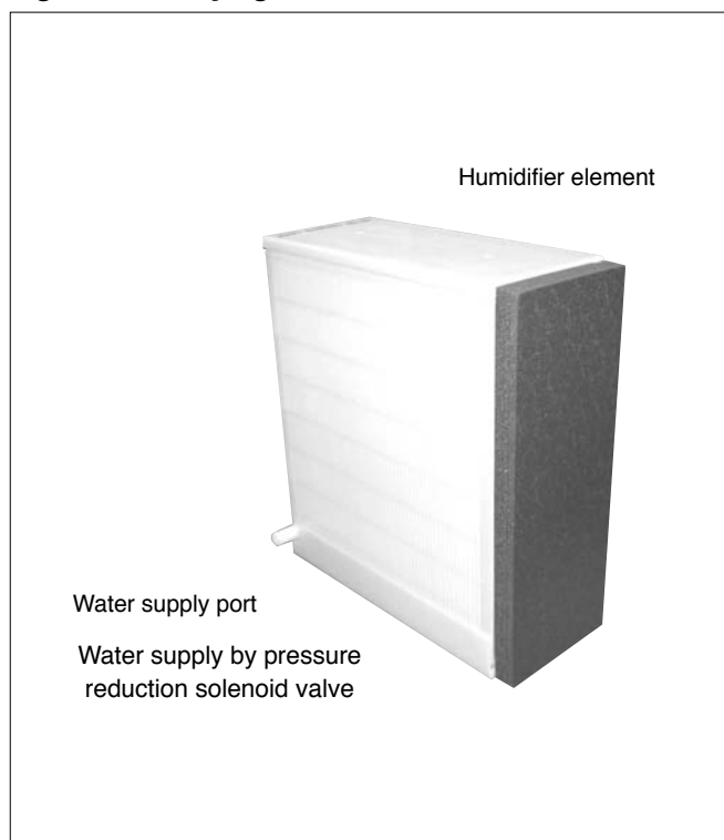
Fig. 2 Humidifying module
