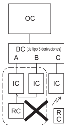
3-1. Funcionamiento agrupado mediante un único controlador remoto
