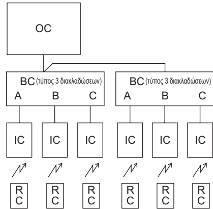
2-3. 2 κουτιά διακλάδωσης (τύπου 3 διακλαδώσεων)
