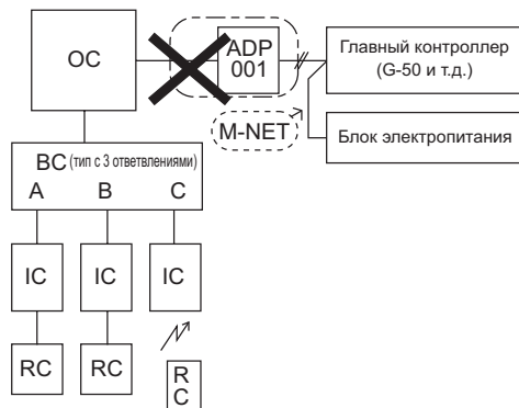
3-3. Подключение адаптера M-NET к наружному
