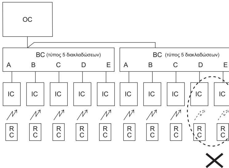
2-4. 2 κουτιά διακλάδωσης (τύπου 5 διακλαδώσεων, 8 εσωτερικές μονάδες κατά μέγιστο)
