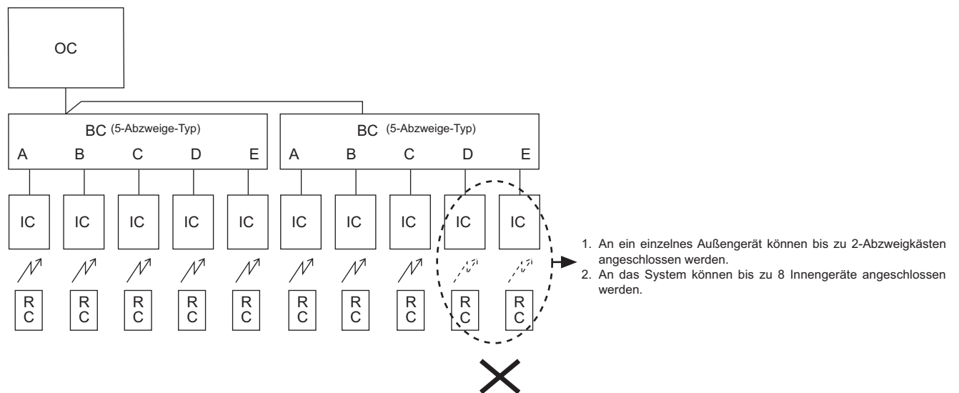
2-4. 2-Abzweigekästen (5-Abzweige-Typ, maximal 8 Innengeräte)
