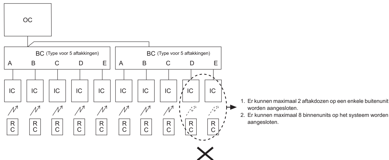
2-4. Aftakdoos met 2 aftakkingen (type voor 5 aftakkingen, maximaal 8 binnenunits)
