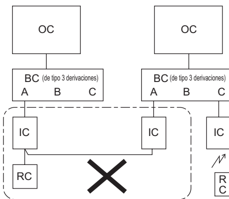
3-2. Funcionamiento agrupado entre distintos sistemas refrigerantes
