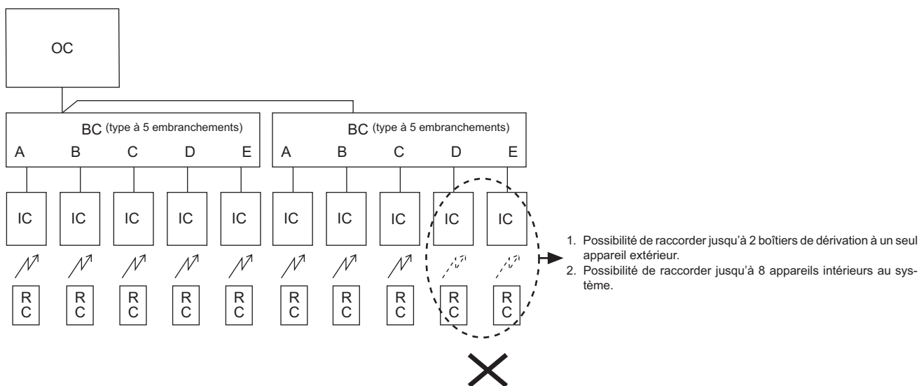
2-4. 2 boîtiers de dérivation (de type à 5 embranchements, 8 appareils intérieurs maximum)
