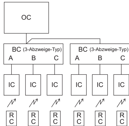
2-3. 2-Abzweigekästen (3-Abzweige-Typ)
