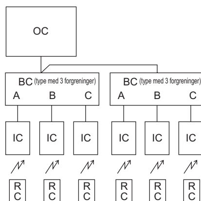
2-3. 2-forgreningsdåser (type med 3 forgreninger)
