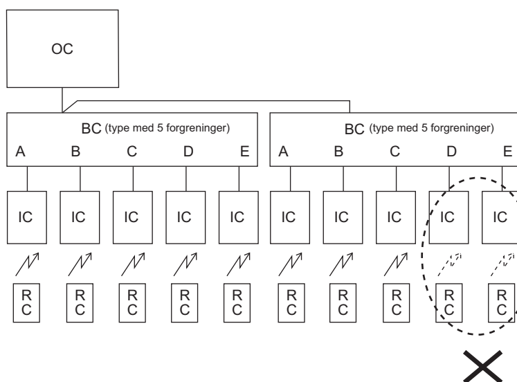
2-4. 2-forgreningsdåser (type med 5 forgreninger, maks. 8 indendørsenheder)
